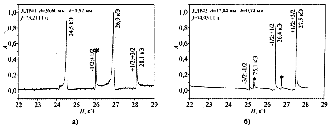
Рис. 3. Собственные спектры ЭСР дисконий рубиновых резонаторов
