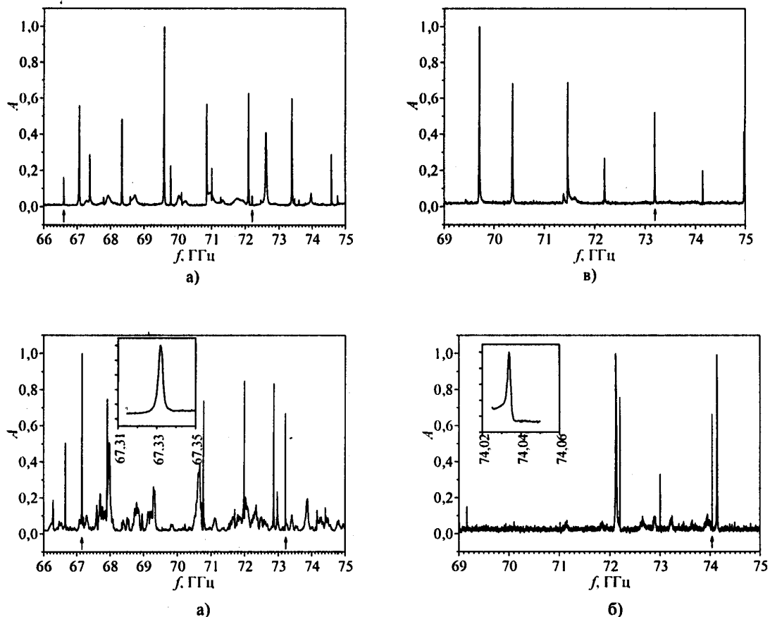
Рис. 2. Спектры ДДР при T = 300\text{ K} (а, в) и T = 4,2\text{ K} (б, г) для обоих резонаторов ДДР#1 (а, б) и ДДР#2 (в, г)
