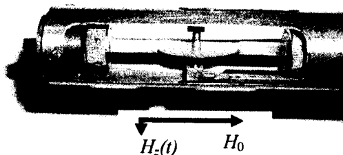
Рис. 1. Резонансная ячейка с рубиновым дисковым диэлектрическим резонатором для исследований эффекта ЭСР в области частот 60-78 ГГц
